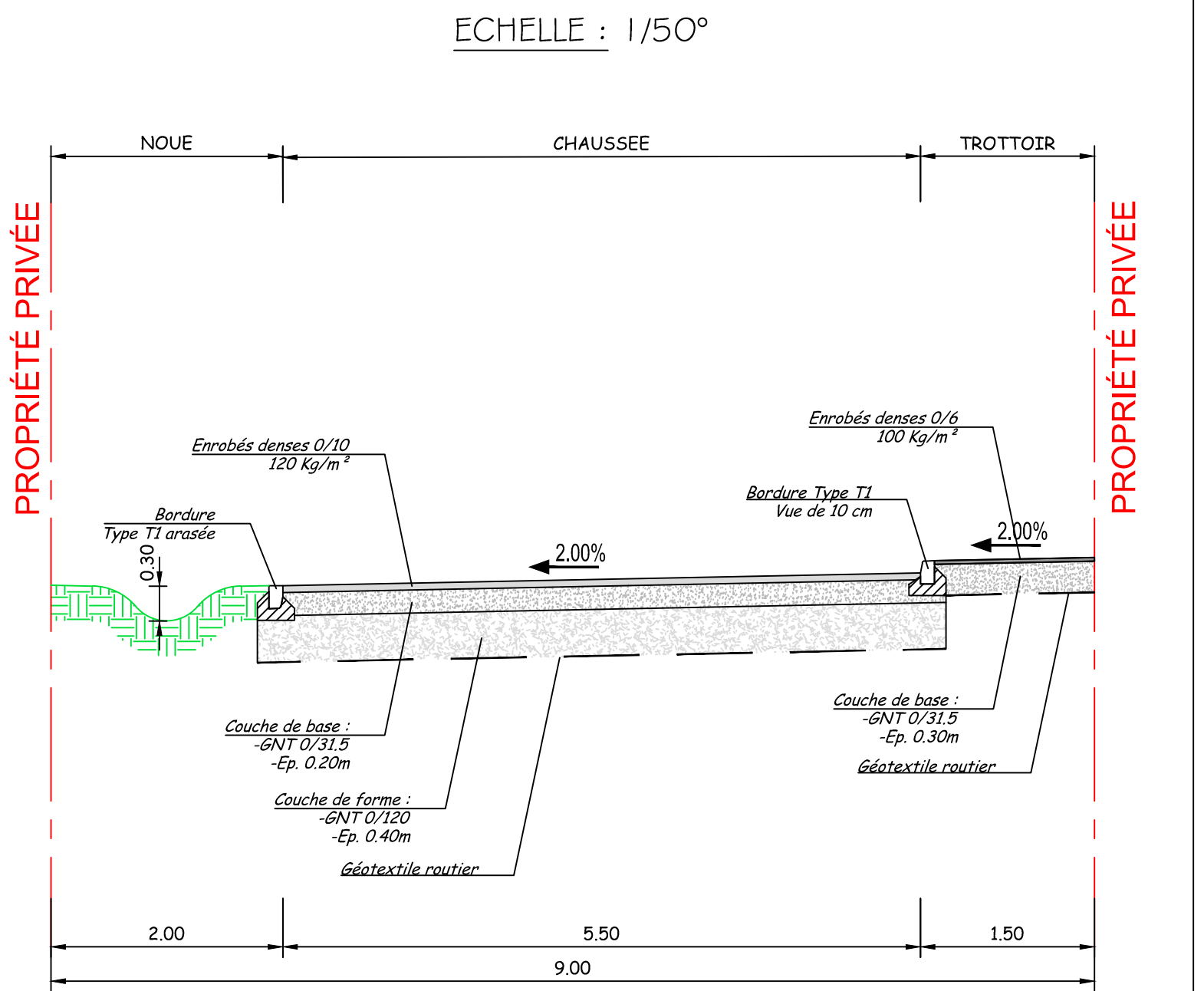
COUPE EN TRAVERS TYPE DD' ECHELLE : 1/50°
