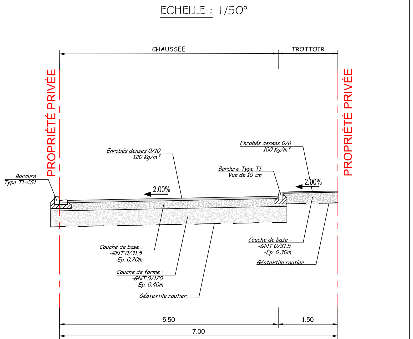
COUPE EN TRAVERS TYPE CC' ECHELLE : 1/50°
