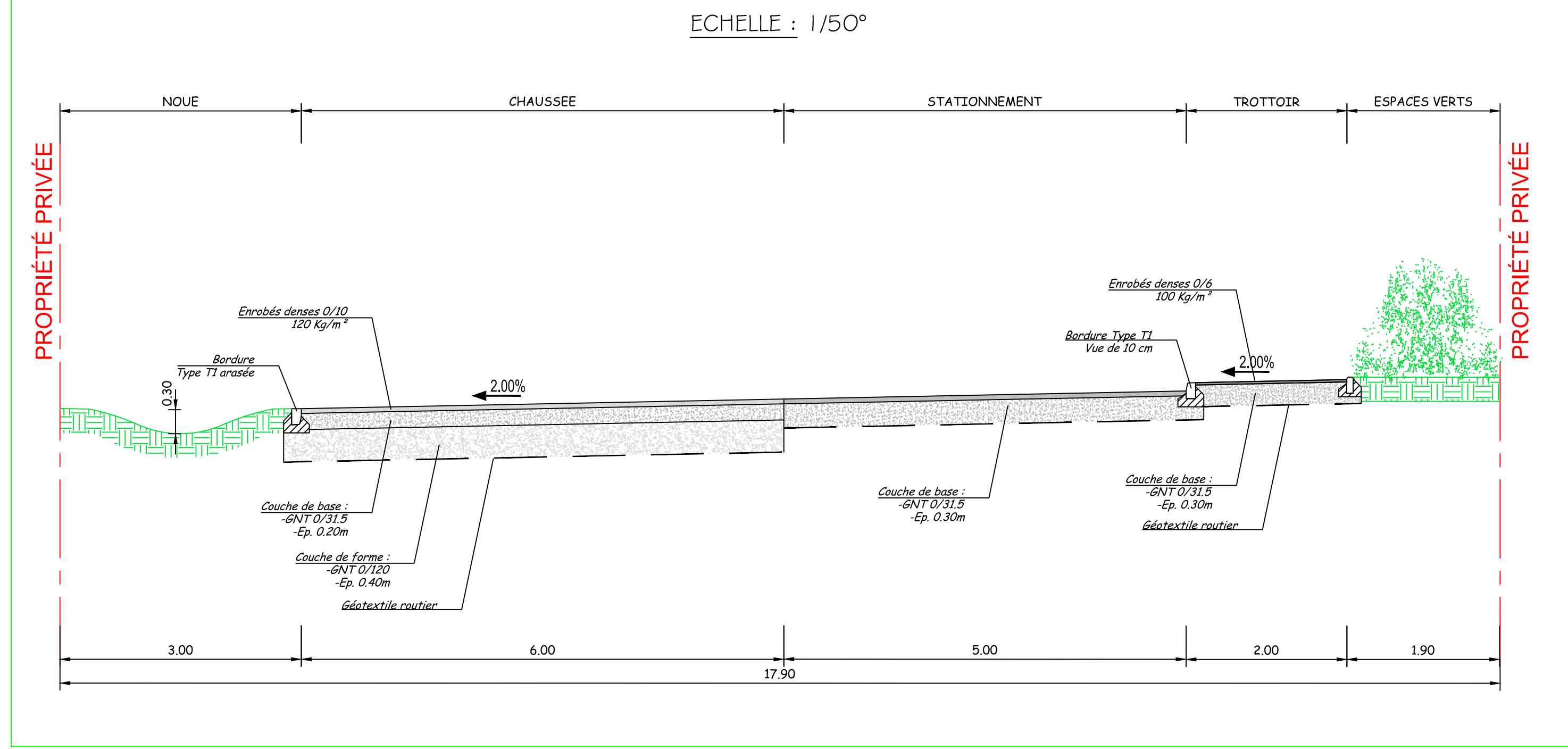
COUPE EN TRAVERS TYPE AA' ECHELLE : 1/50°
